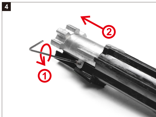
移除槍機頭外罩。 Remove the Bolt Head.
