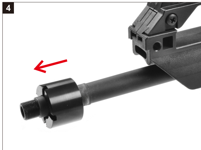
移除槍管固定環。 Remove the Barrel Screw
